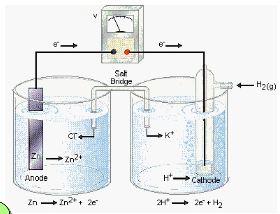
Schema pila Daniell (cella elettrochimica) VARIANTI
